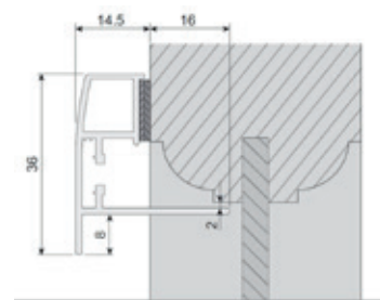
FrameFix™, ram
