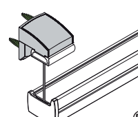
Plastvinkel, 5 mm avstånd - uppspända modeller, endast 20/25 mm.
