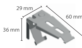
CHR överlist 64 mm
