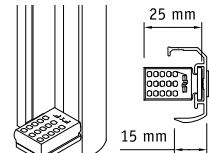
* Till modell 3242 får man en kort vinkel, där beslag/wirefot monteras. Här visas wirefot.
